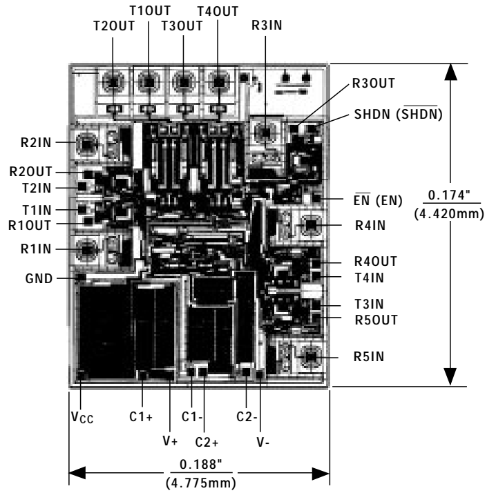
MAX211E/MAX213E/MAX241E
